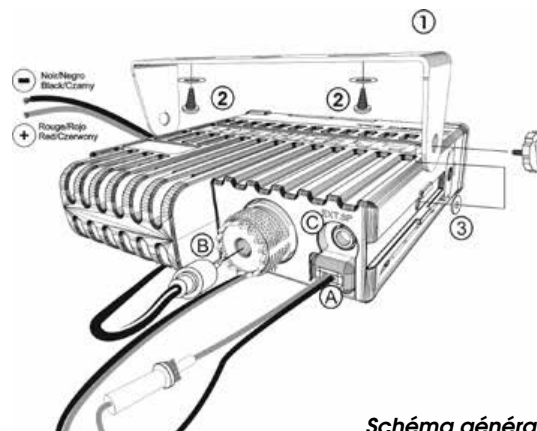
Schéma général de montage
